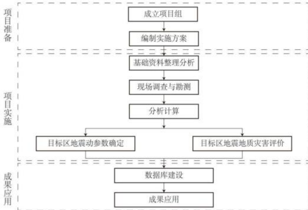
图1 区域性地震安全性评价工作流程
