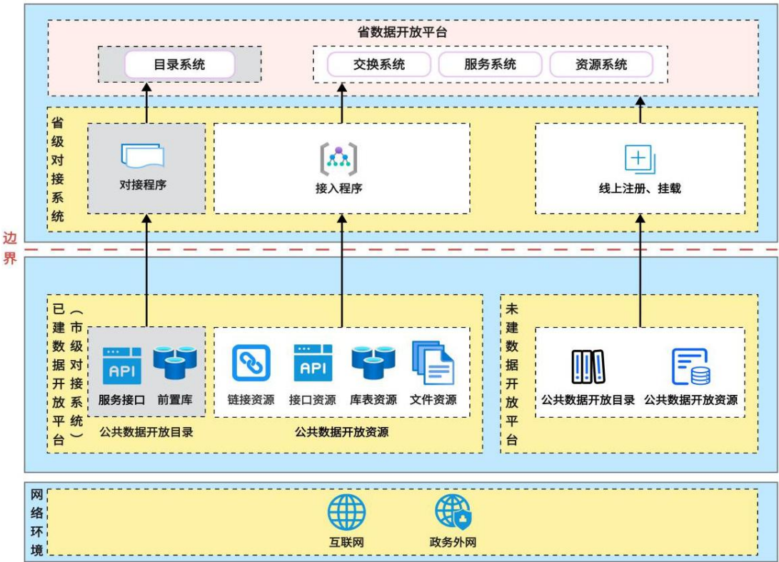
图 1 接入总体框架示意图
