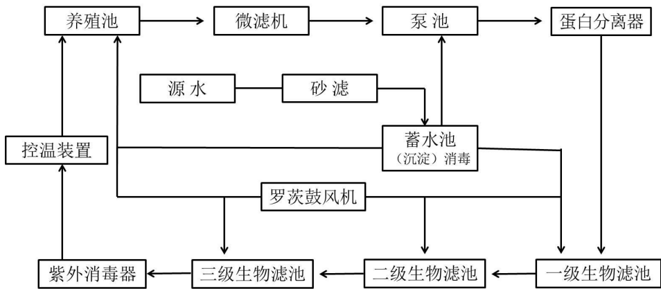
图 1 欧洲舌齿鲈亲鱼循环水养殖系统工艺流程图
