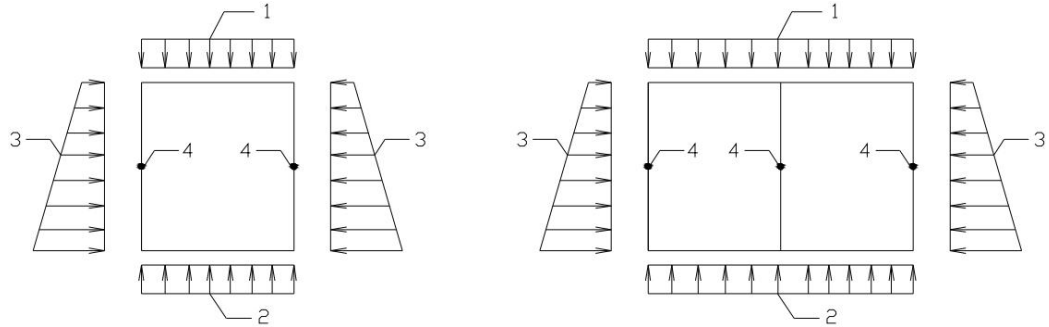
1-综合管廊顶板荷载；2-综合管廊地基反力；3-综合管廊侧向水土压力；4-拼缝接头旋转弹簧
