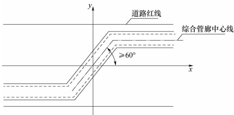
图 4 综合管廊最小交叉角示意图
