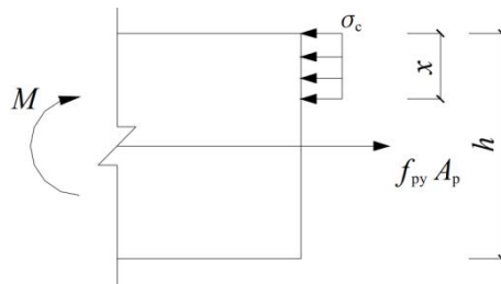
图 9.5.8 接头受弯承载力计算简图
