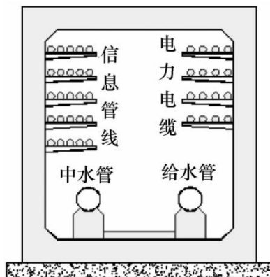
图8 断面示意图4
