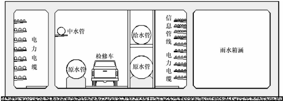
图 5 断面示意图 1
