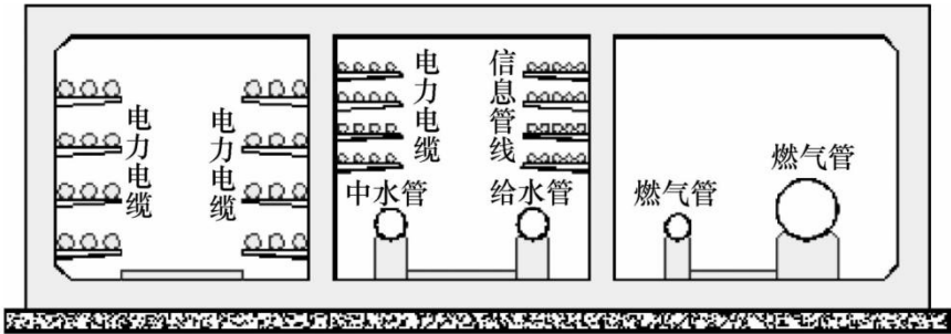
图 6 断面示意图 2
