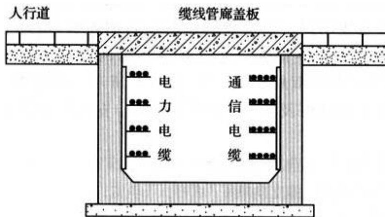
图3 缆线综合管廊示意图
