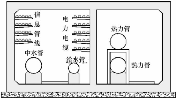
图 7 断面示意图 3
