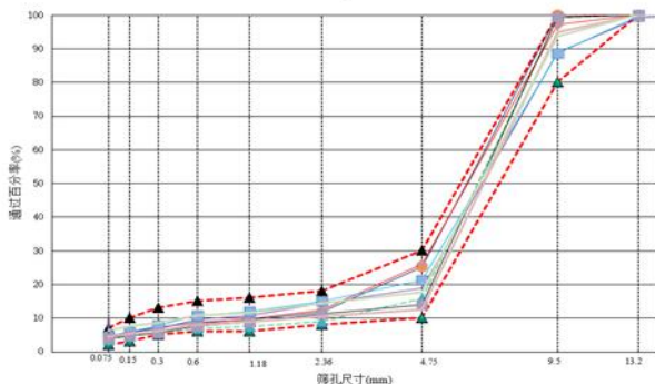
图 C.2 辽宁阜锦高速 FRAS12 (5mm~10mm) 级配 监测数据
