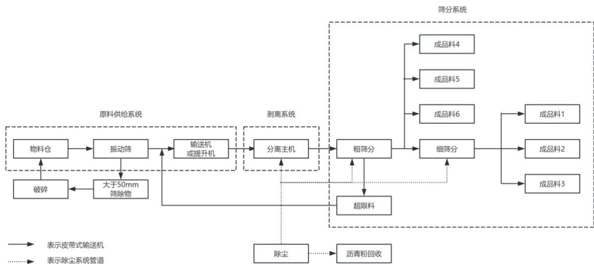
图 1 精细加工工艺流程示意图
