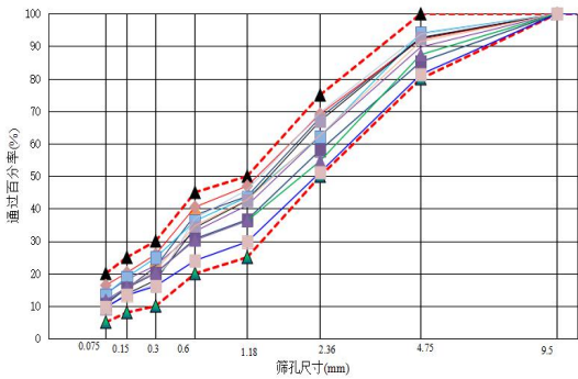
图 C.1 辽宁阜锦高速 FRAS15 (0mm~5mm) 级配 监测数据
