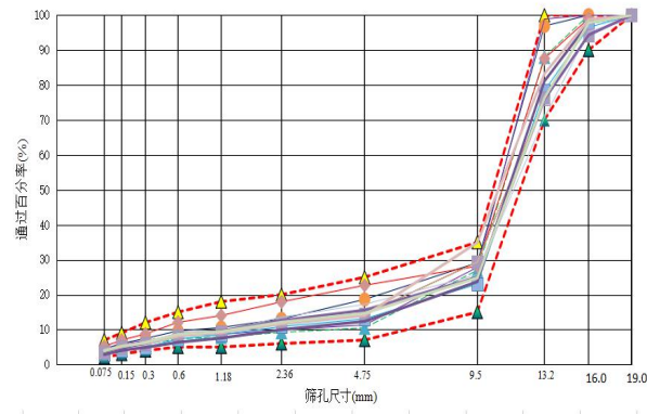
图 C.3 辽宁阜锦高速 FRS10（10mm~15mm）级配监测数据
